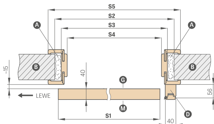
SP1Nz nebo SP1Nb (levý verze přední)
