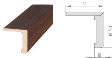
ÚHELNÍK S PRODLOUŽENÝM JAZÝČKEM K NASTAVITELNÉ ZÁRUBNI
